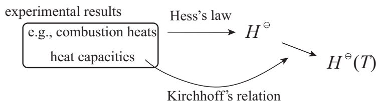
Figure 25.2: どうやって標準エンタルピーを測定できる量から決めるか; まとめの \Delta H は加法的である. これが Hess の法則 Hess's law である. 次の反応熱は測定で
