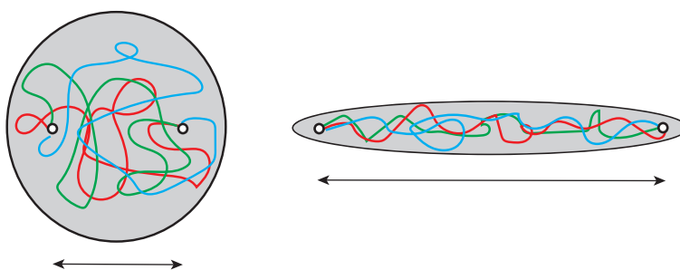
Figure 21.3: 引き延ばされると鎖の動ける範囲が少なくなる。3色違うコンフォメーションが描いてあり、大体の動ける範囲が灰色の領域。
